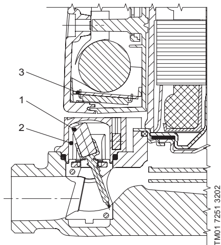
Рис. 1 Разрез внутреннего реле потока, UPA 15-90(N)
